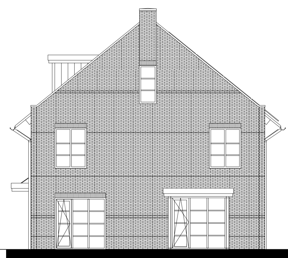
Zijgevel (1:100)
