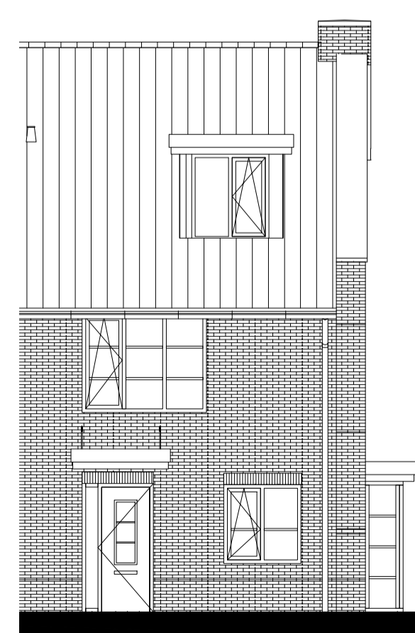
Voorgevel (1:100)
