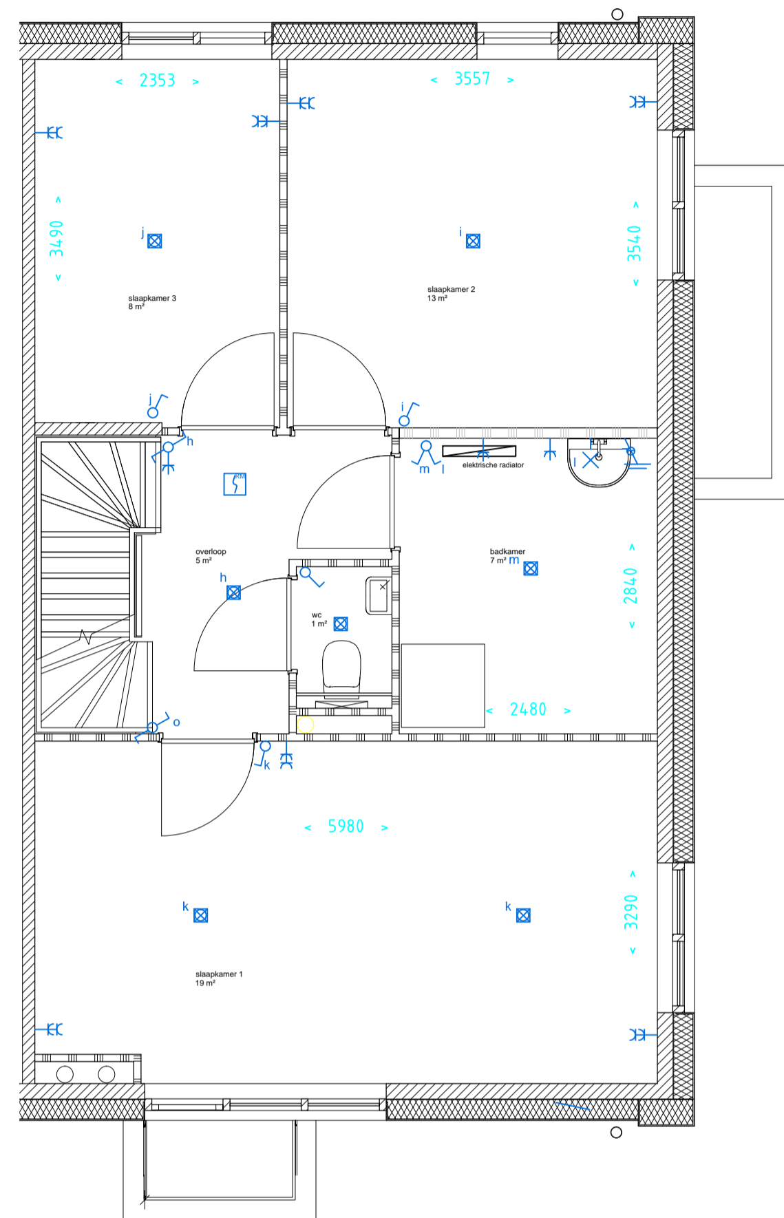
1e verdieping (1:50)
