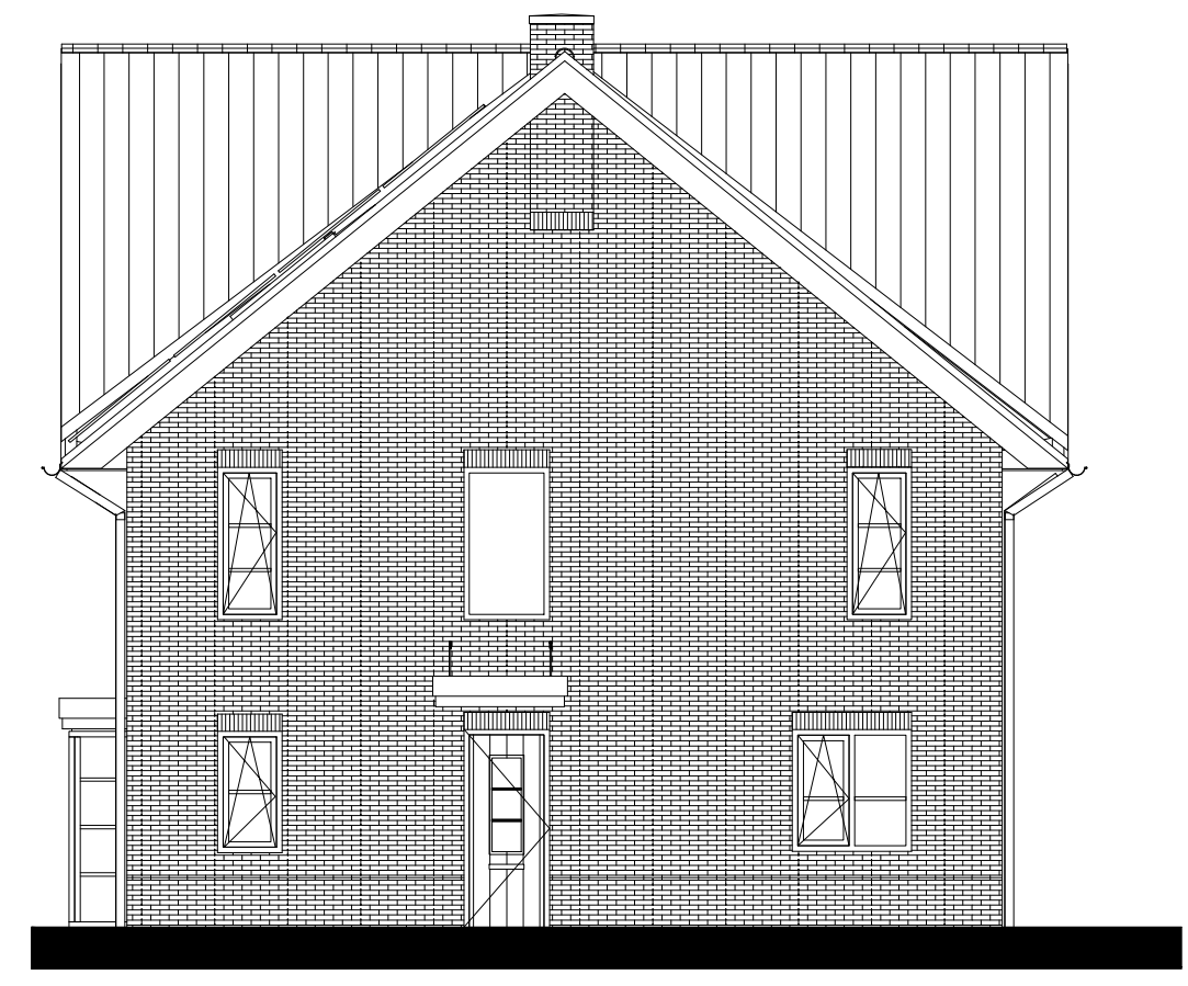
Zijgevel (1:100)
