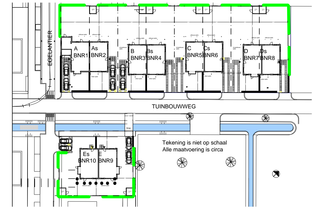
Situatie (1:750)
