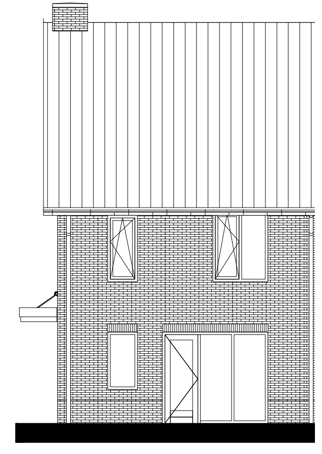
Achtergevel (1:100)
