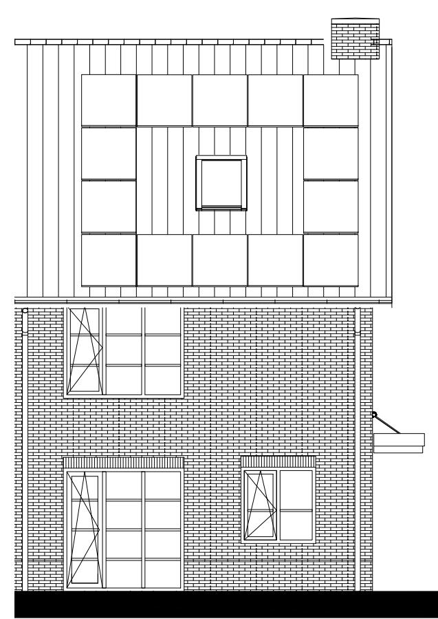
Voorgevel (1:100)
