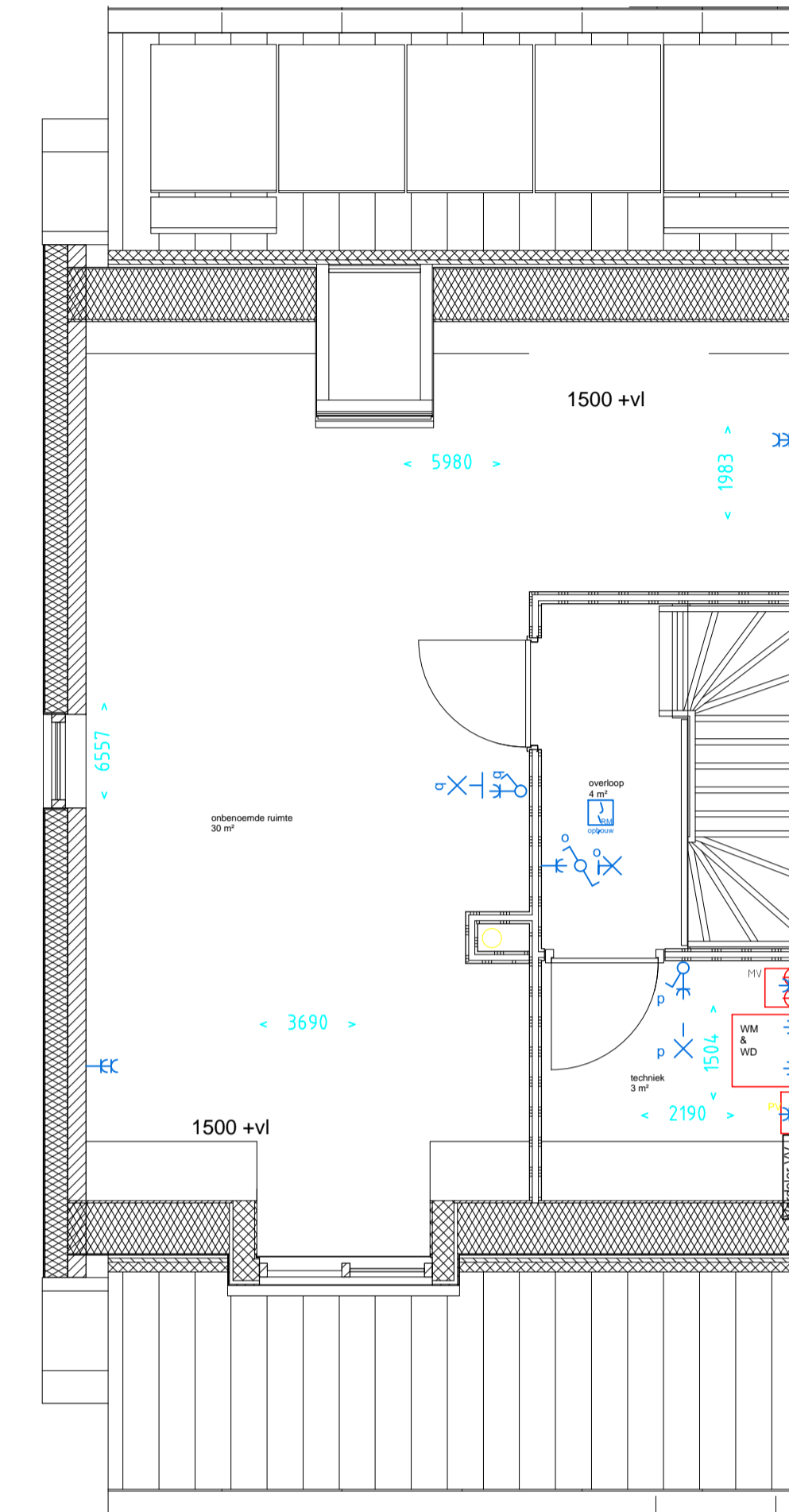
2e verdieping (1:50)
