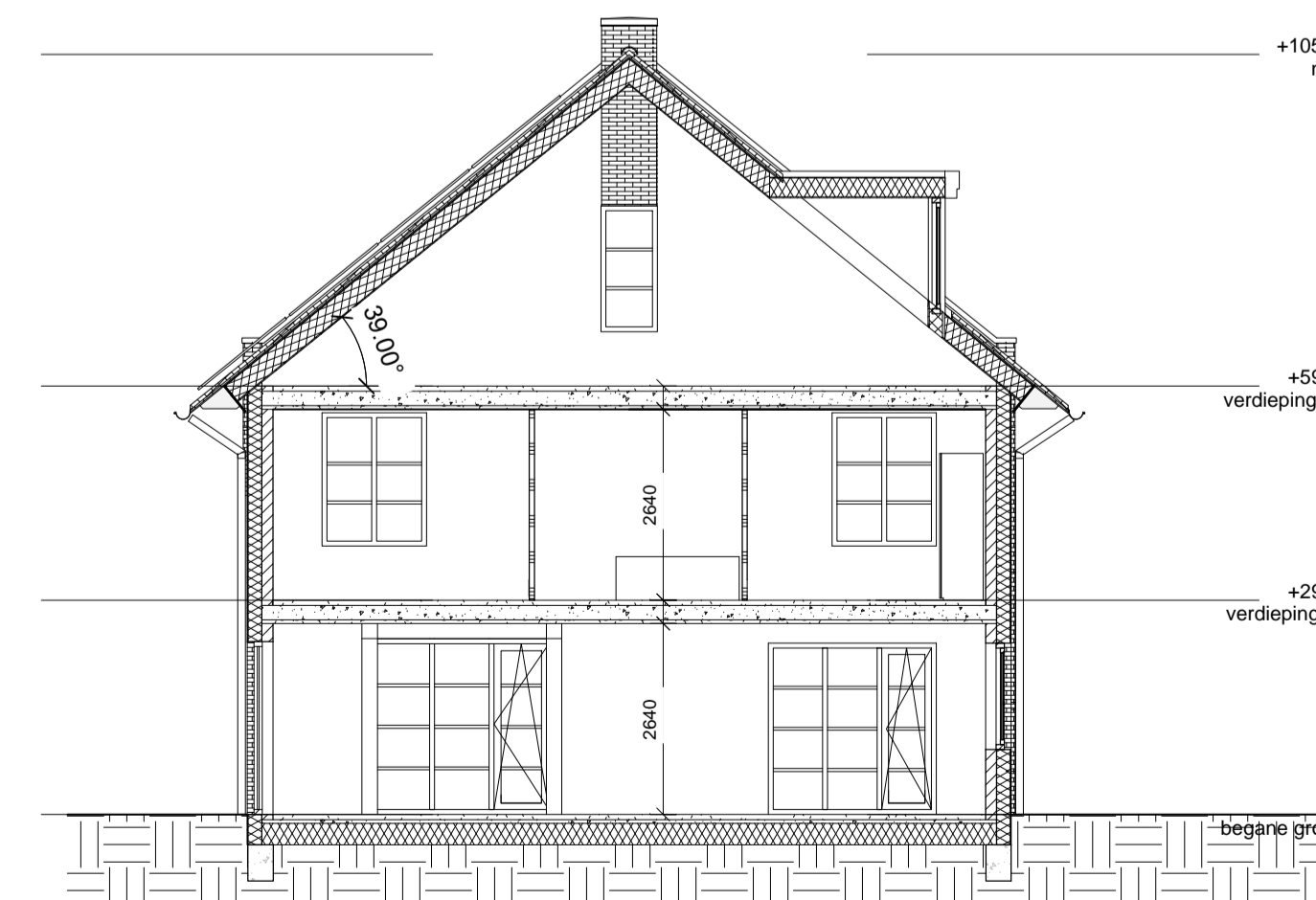
Doorsnede (1:100)
