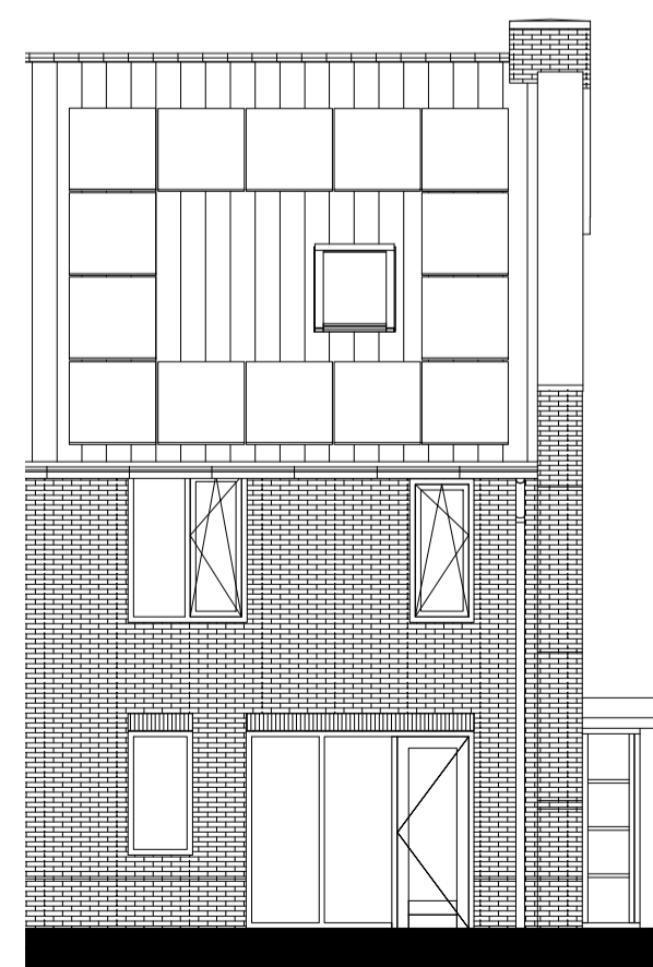
Achtergevel (1:100)
