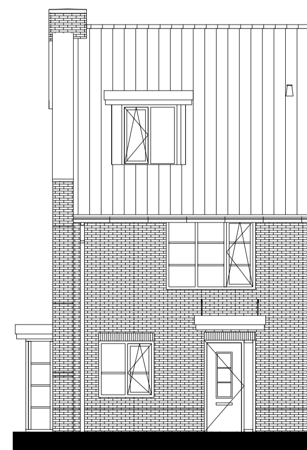
Voorgevel (1:100)
