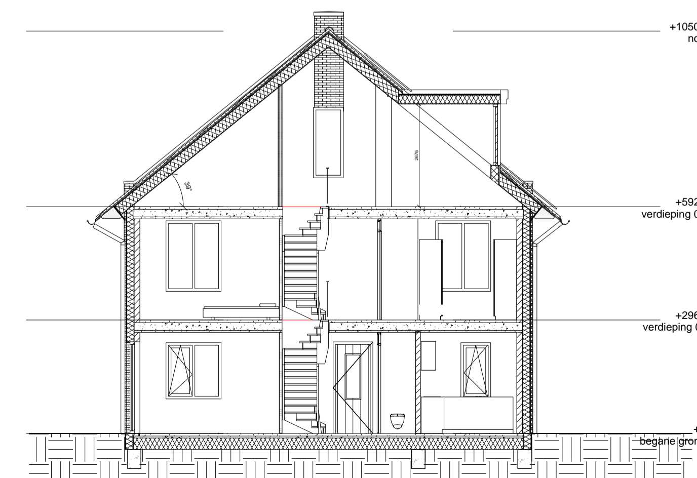
Doorsnede (1:100)
