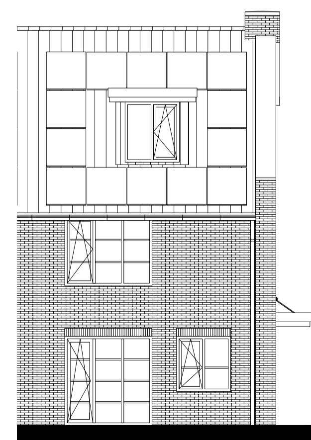
Voorgevel (1:100)
