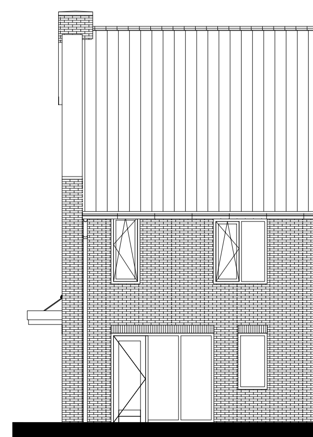
Achtergevel (1:100)
