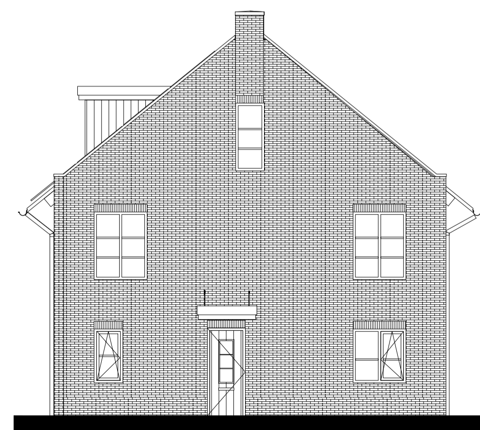
Zijgevel (1:100)
