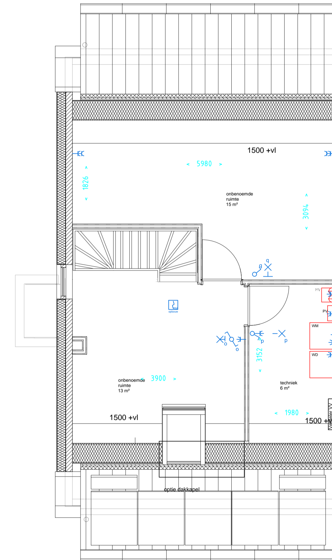
2e verdieping (1:50)
