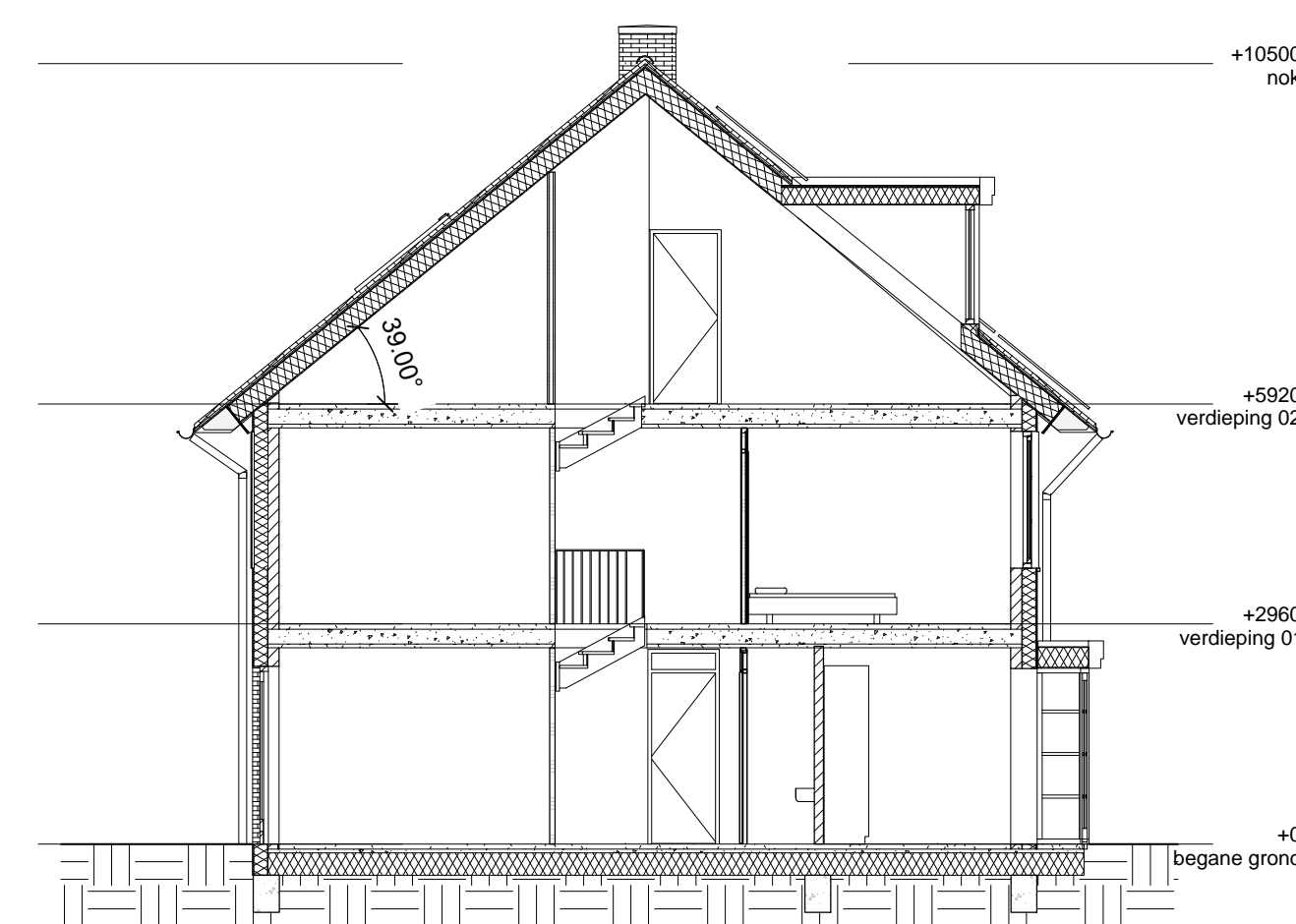
Doorsnede (1:100)
