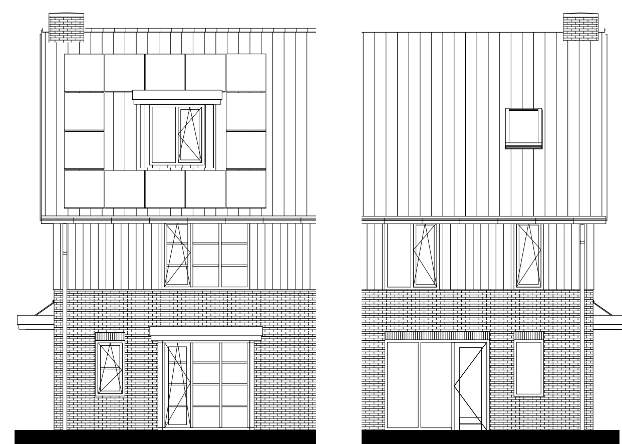
Voorgevel (1:100)
