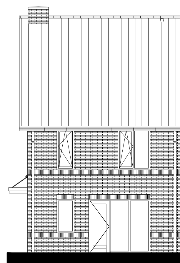
Achtergevel (1:100)
