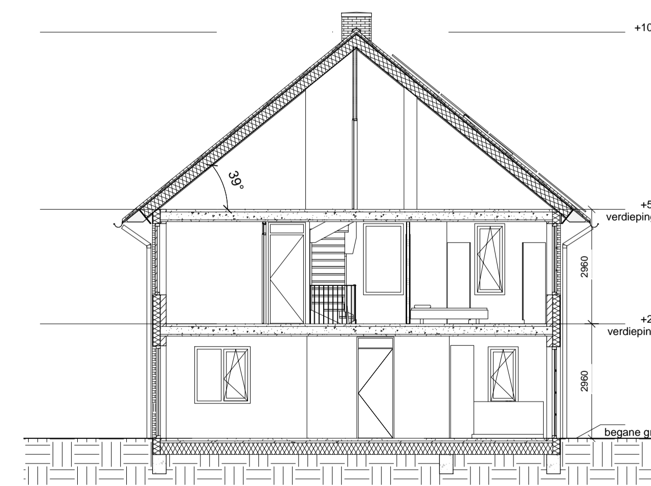
Doorsnede (1:100)
