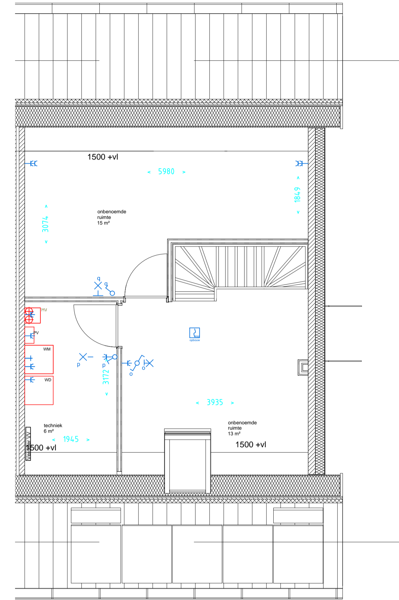
2e verdieping (1:50)
