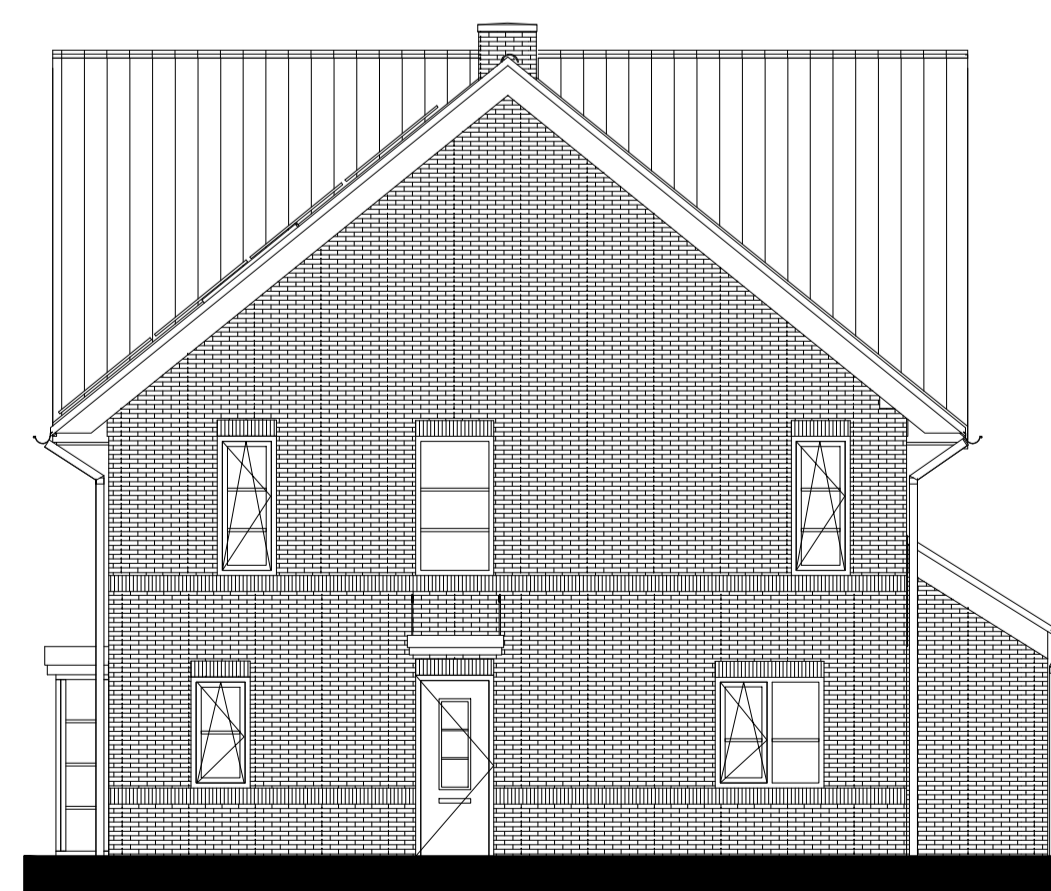
Zijgevel (1:100)
