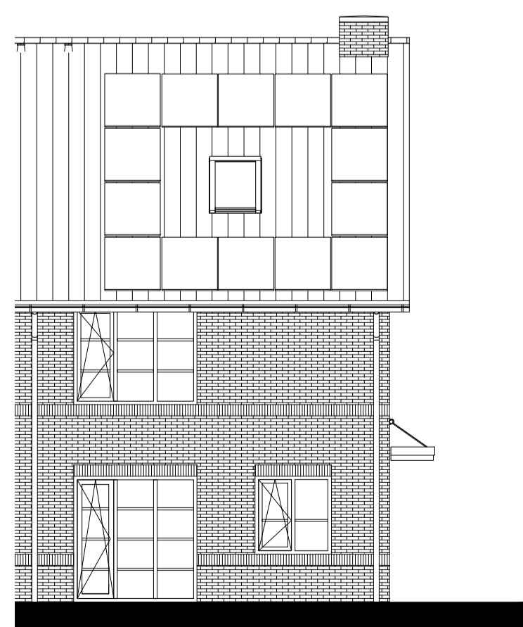
Voorgevel (1:100)
